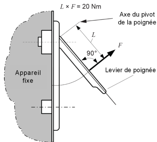
a) Poignée de type levier plat
