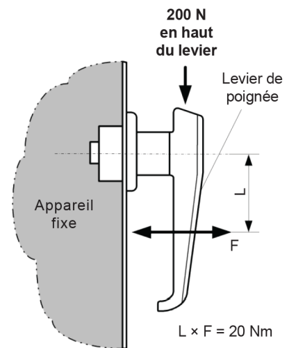
b) Poignée de type levier
