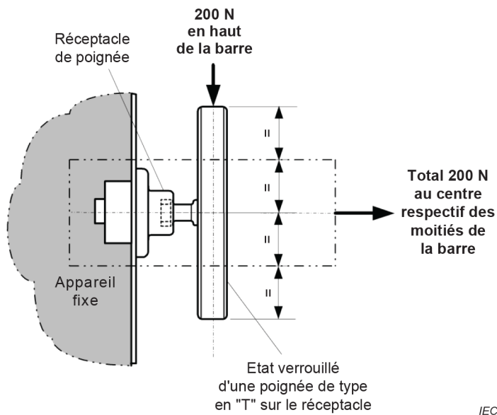
c) Poignée de type en "T"
